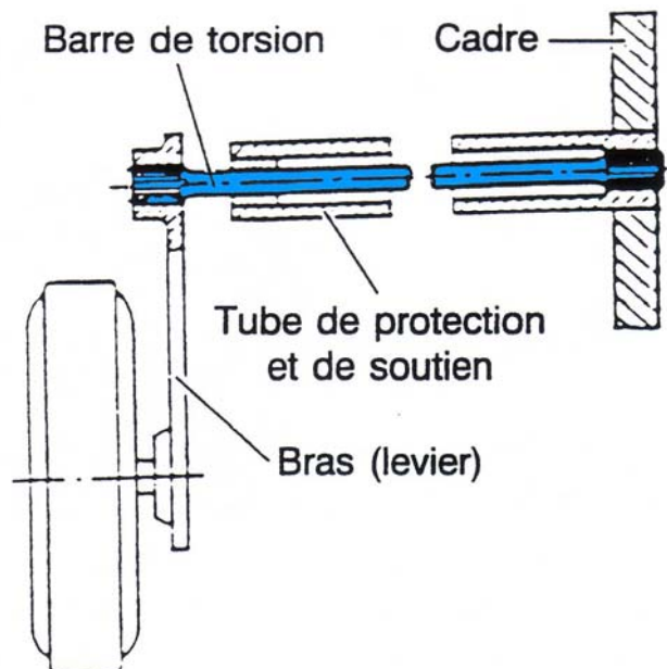
Barre de torsion
